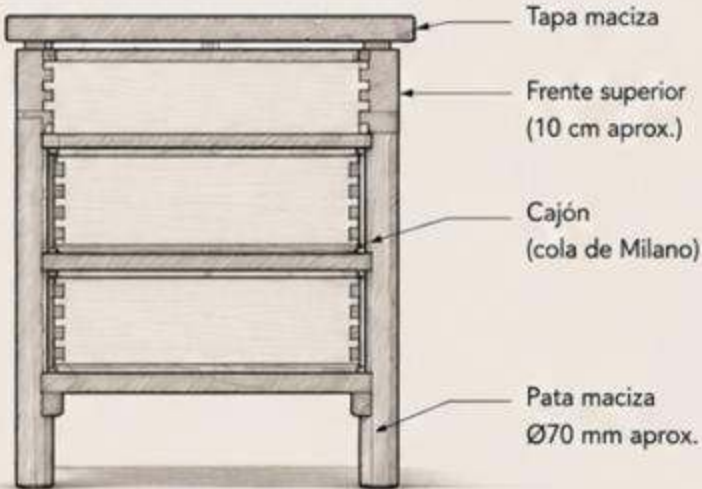
CORTE FRONTAL
