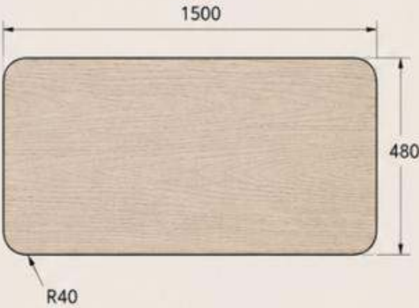
PLANTA
