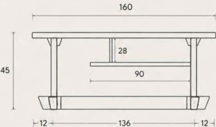
VISTA FRONTAL (técnica)
