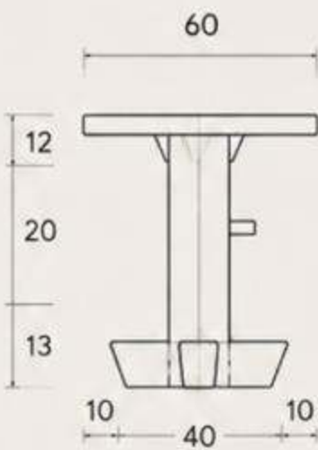
VISTA LATERAL (técnica)
